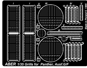
ABER 1/35 Grills for Panther, Ausf.G/F
