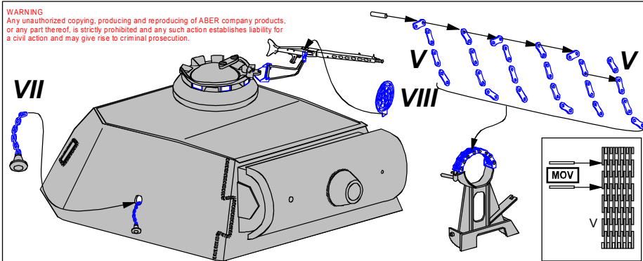
ABER 1/35 Grills for Panther, Ausf.G/F
